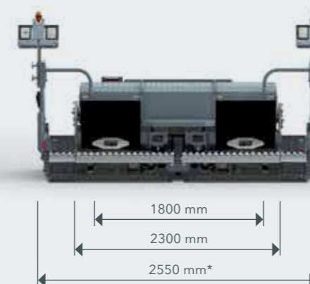
Transporte sencillo con extensiones mecánicas de 25 cm
